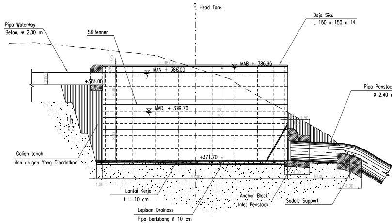
POTONGAN MELINTANG
