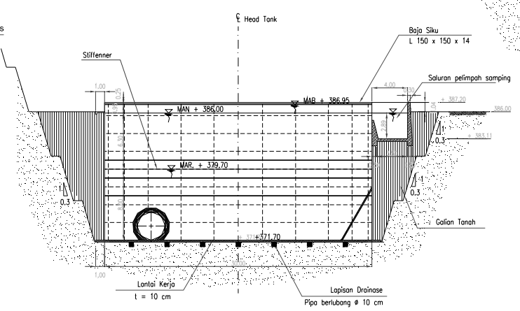
POTONGAN MELINTANG PELIMPAH
