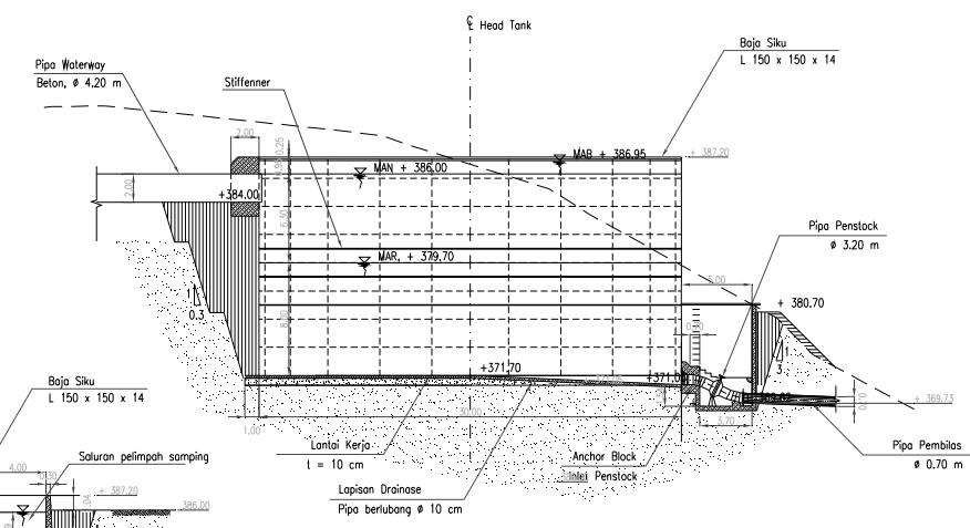
POTONGAN MELINTANG PEMBILAS
